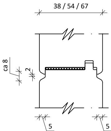
LX stapeldorpel / tussenstijl detail
