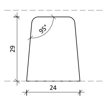
Horizontale lat
