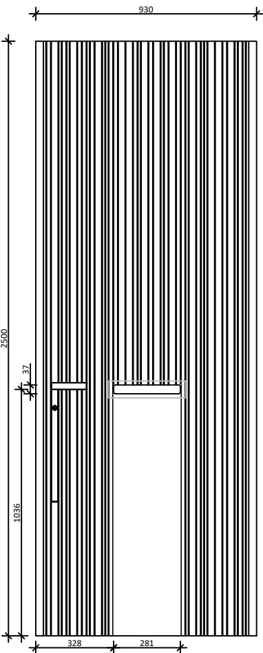
Hoog model 2401 - 2600
