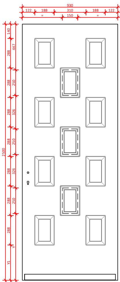
Hoog model 2401 - 2600
