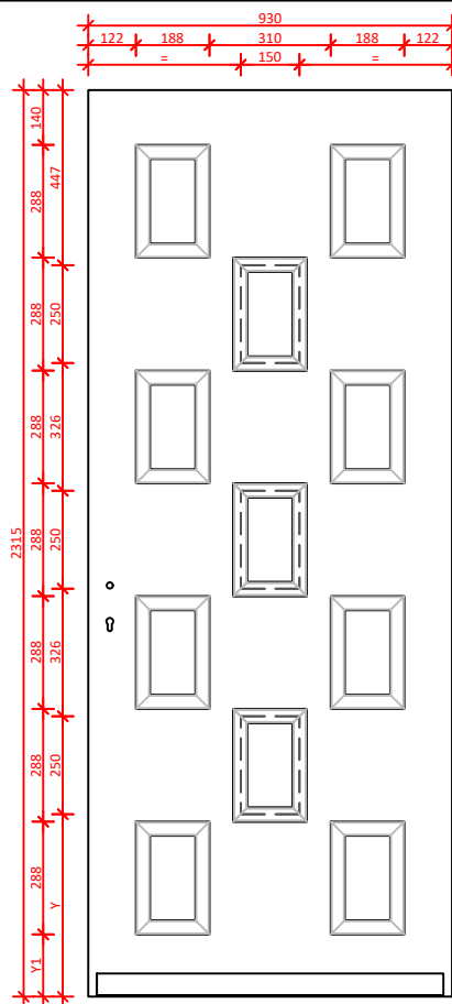
Midden model 2201 - 2400
