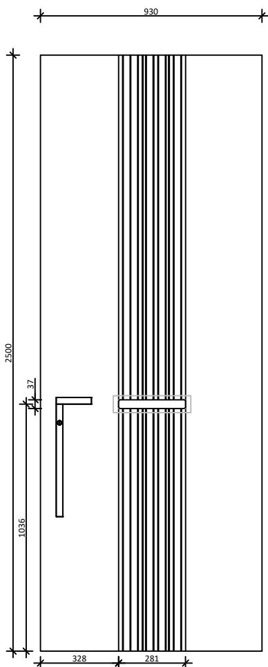
Hoog model 2401 - 2600
