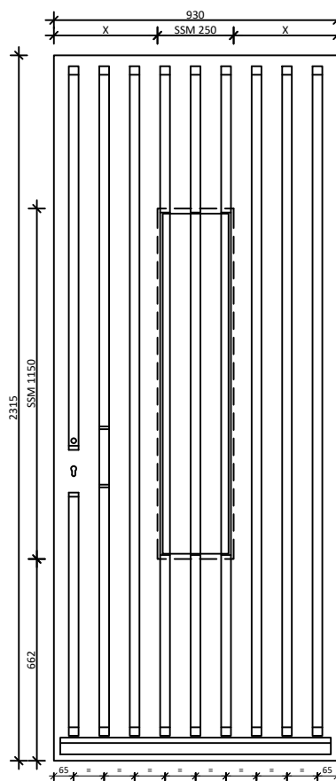
Midden model 2201 - 2400
