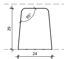
Horizontale lat
