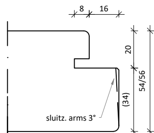
54-04: 34-16 Kader-profilering (voor renovatie)
