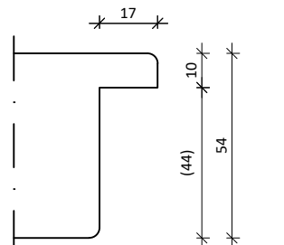
Contraspionning 17x44 passieve deur van 54-S01 deurstel
