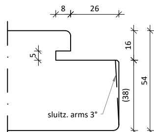
54-07: 38-26 Kader-profilering (voor 25mm kozijnsponning)
