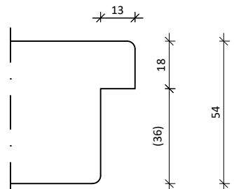
Contraspionning 13x36 passieve deur van 54-S04 deurstel
