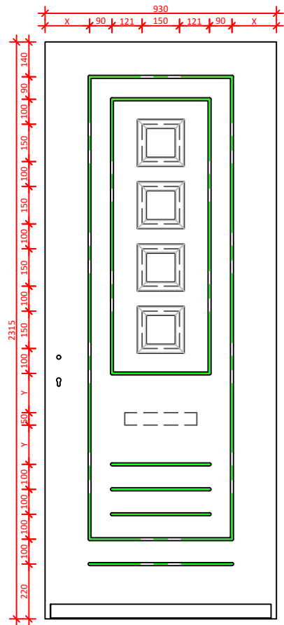
Groeven 12 mm Midden model 2201 - 2400
