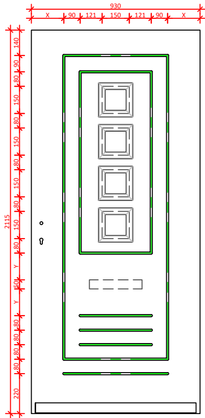
Groeven 12 mm Laag model 1900 - 2200
