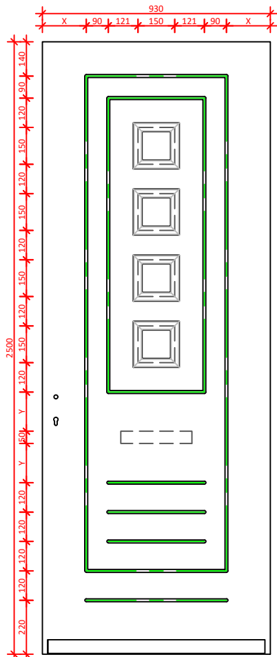
Groeven 12 mm Hoog model 2401 - 2600
